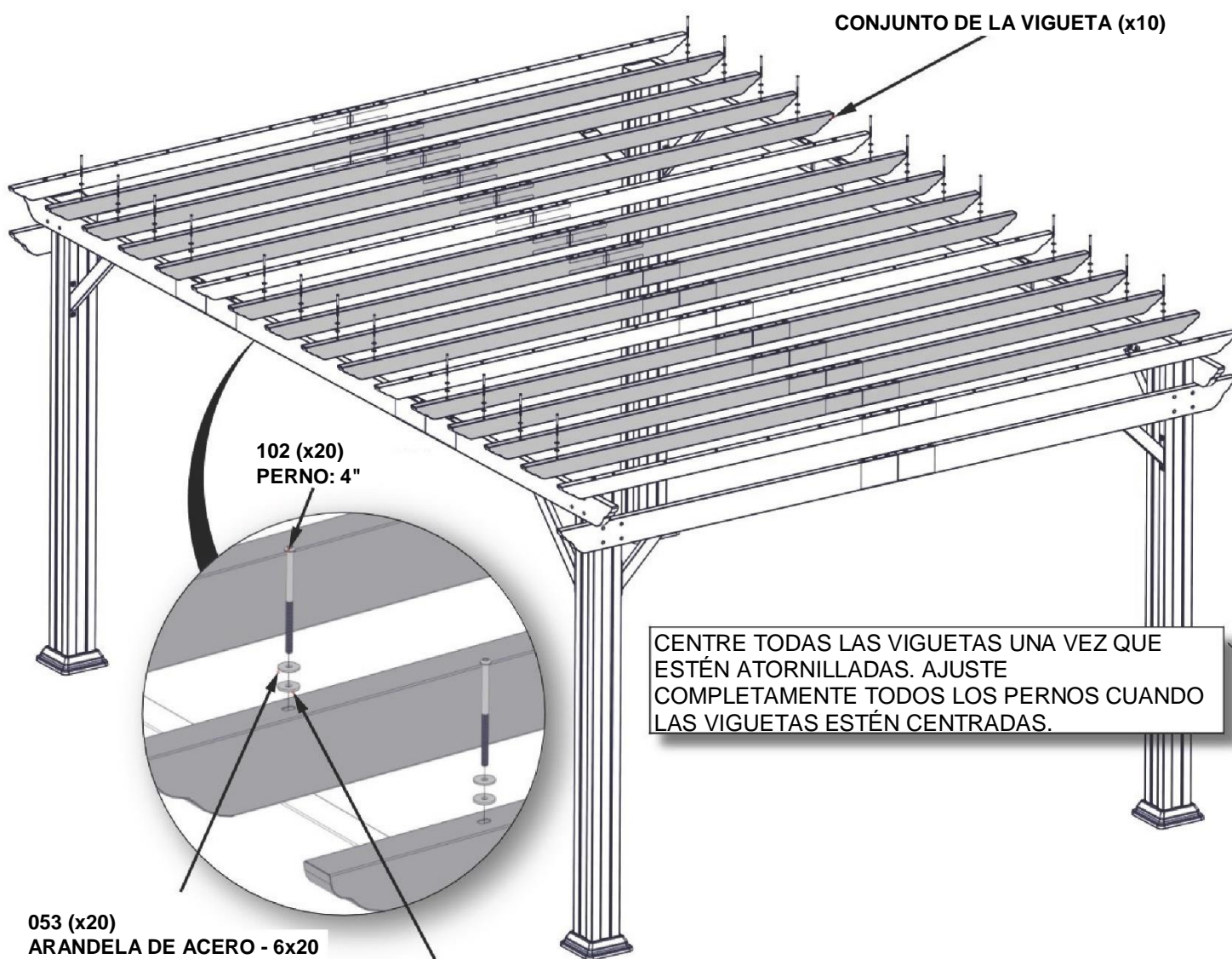
054 (x20) ARANDELA SELLADORA
