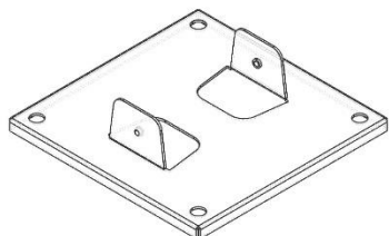
G1 (4) | PLACA PARA PIE DE POSTE - A4M01278
