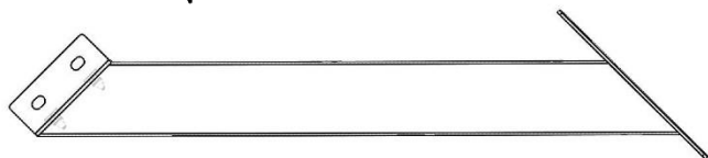
F2 | SOPORTE ANGULAR LARGO - A4M01274 (2) | 1 1/8" x 4" x 21 1/2" (30 x 101 x 546)
